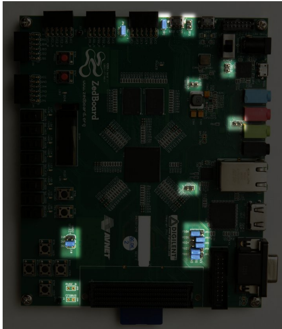
Zedboard 上突出显示的跳线设置
